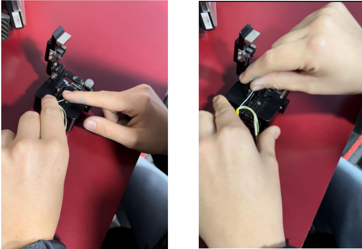
Figura 55. Proceso de corte de fibra óptica.
