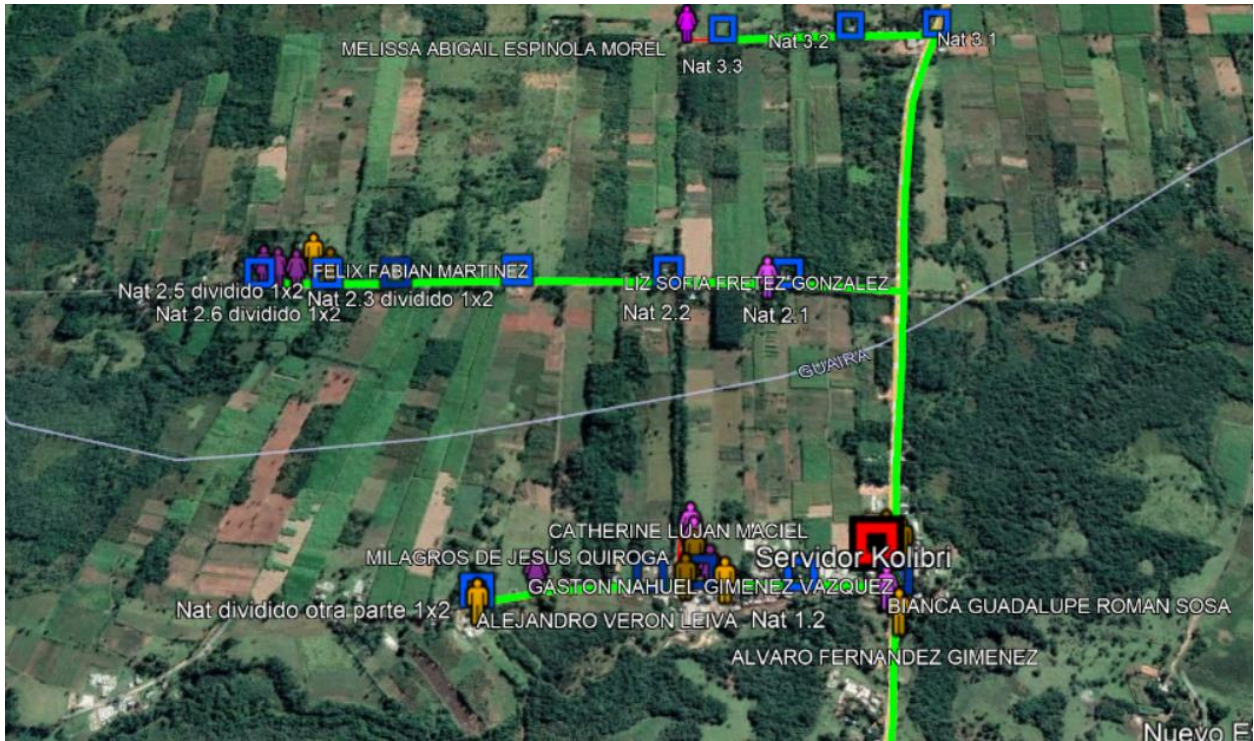
Figura 58. Croquis-Implementación Kolibri.
